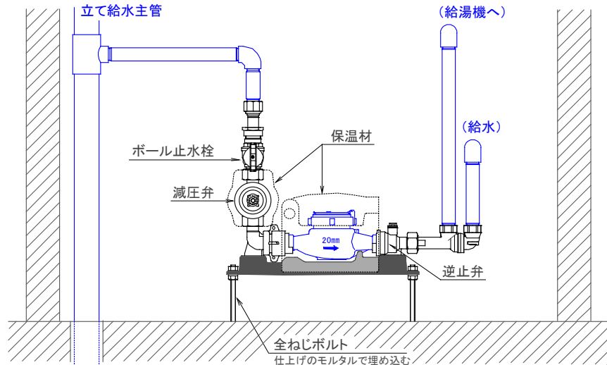
【図-14. 2. 1 パイプシャフト内配管 参考模式図】
